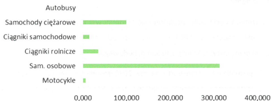
Rysunek 8. Zestawienie łącznej wielkości emisji CO 2 pojazdów z podziałem na rodzaj pojazdu w roku 2000.
