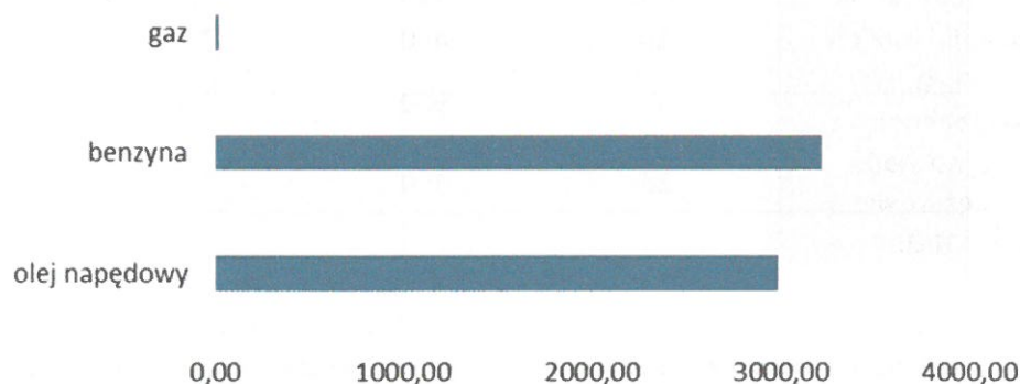
Rysunek 9. Zestawienie łącznej wielkości emisji CO 2 pojazdów z podziałem na rodzaj zużywanego paliwa w roku 2013.
