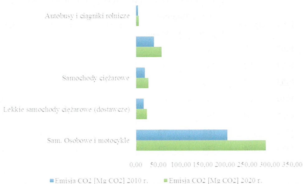
Rysunek 10. Emisja CO 2 z transportu z podziałem na poszczególne pojazdy, na rok 2010 z prognozą na 2020.
