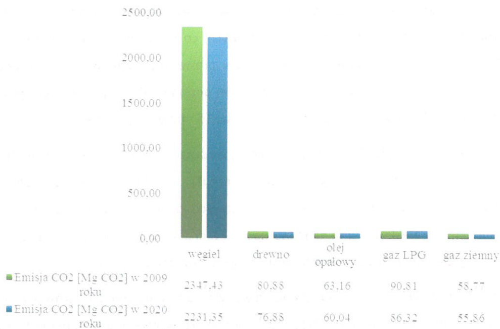
Rysunek 21. Emisja CO 2 [Mg CO 2 ] - handel, usługi, przemysł, w roku 2009 i 2020.
