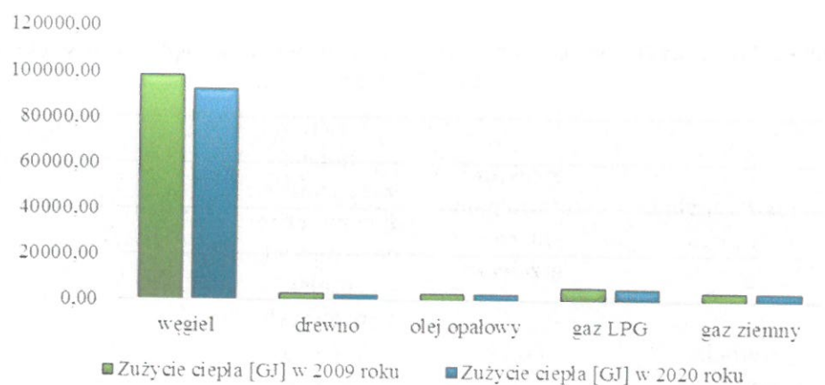
Rysunek 18. Zużycie poszczególnych paliw na cele grzewcze - mieszkalnictwo.
