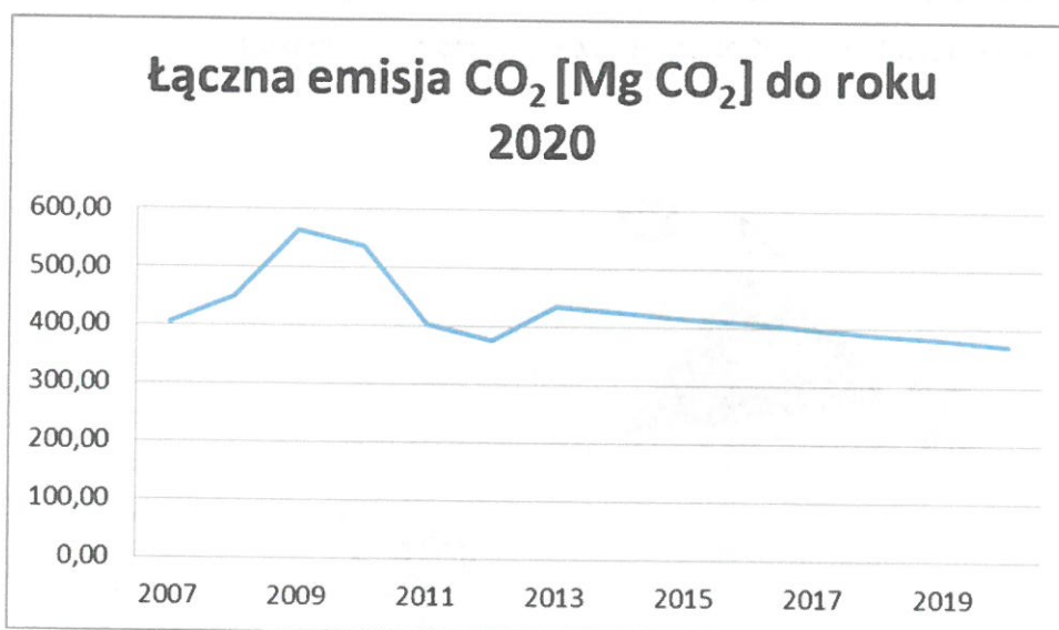
Rysunek 12. Łączna emisja CO 2 [Mg CO 2 ] ze zużycia paliw gazowych do roku 2020.
