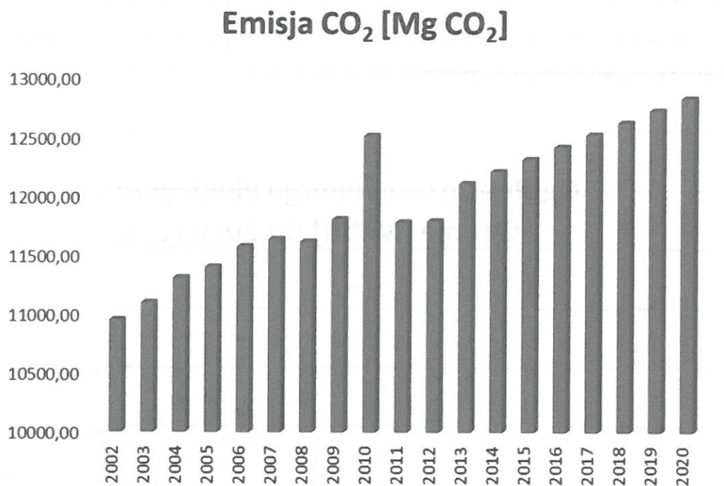
Rysunek 15. Emisja CO 2 [Mg CO 2 ] do roku 2020.
