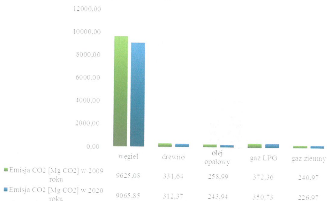
Rysunek 19. Emisja CO 2 [Mg CO 2 ] - mieszkalnictwo, porównanie emisji w roku 2009 i 2020.
