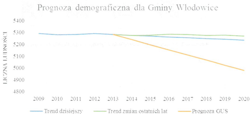
Rysunek 2. Prognozowane zmiany demograficzne do roku 2020.
