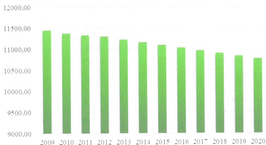
Rysunek 17. Prognoza emisji CO 2 [Mg CO 2 ] - mieszkalnictwo.
