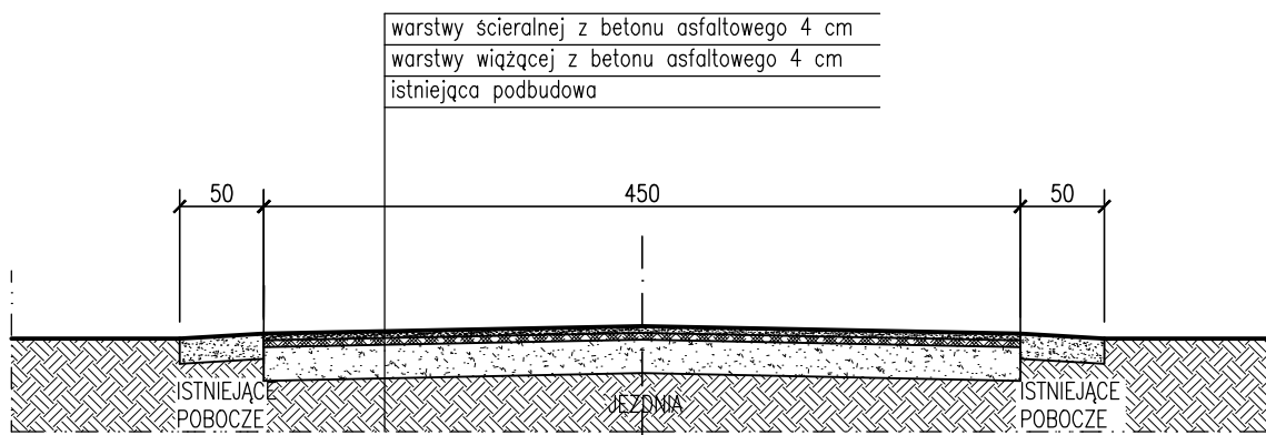
PRZEKRÓJ POPRZECZNY JEZDNI
