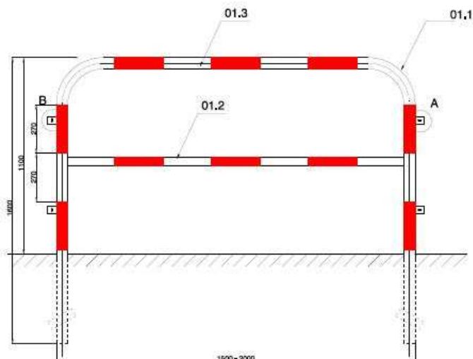
Rys. 1. Wzór bariery ochronnej z rur stalowych U-12 a
